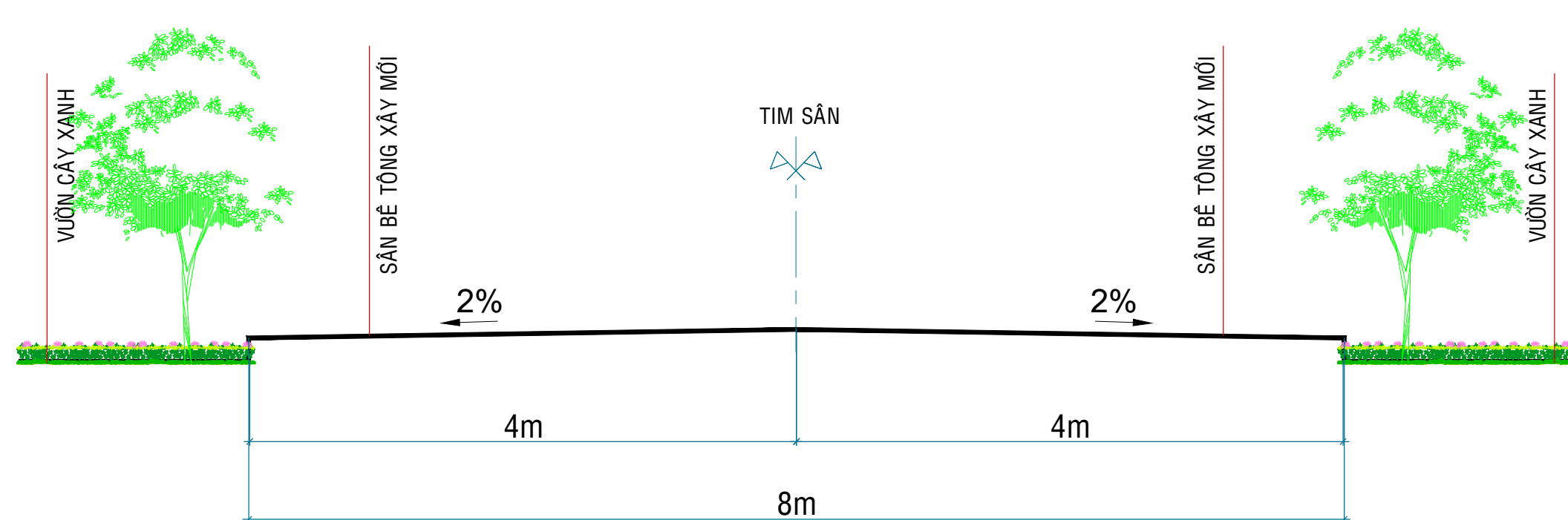
MẶT CẮT ĐƯỜNG VÀO LÀM MỚI
