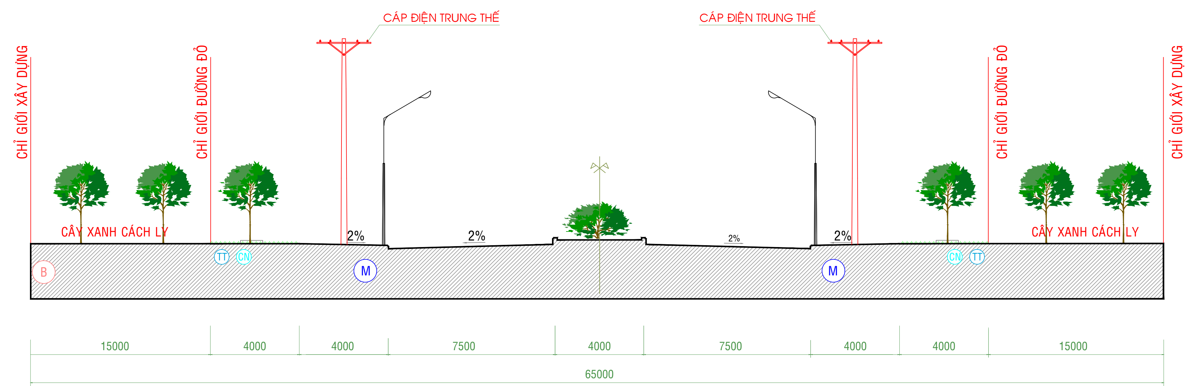
MẶT CẮT NGANG ĐƯỜNG N2
