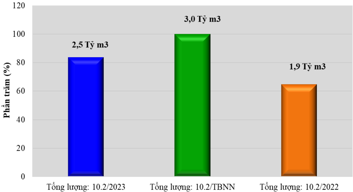
Hình 3. Tổng lượng dòng chảy tại trạm Chiềng Sên trong nửa cuối tháng 10/2023
