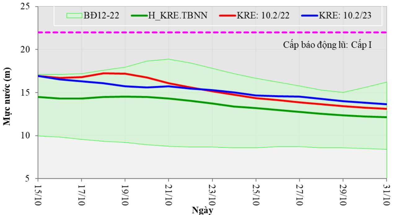
Hình 4. Diễn biến mực nước tại trạm Kra-chê trong nửa cuối tháng 10/2023
