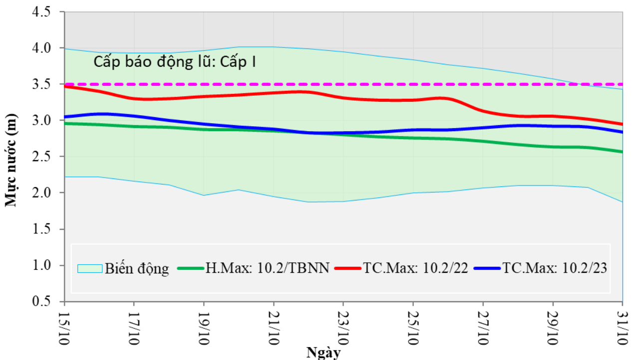
Hình 9. Diễn biến mực nước lớn nhất ngày tại trạm Tân Châu nửa cuối tháng 10/2023
