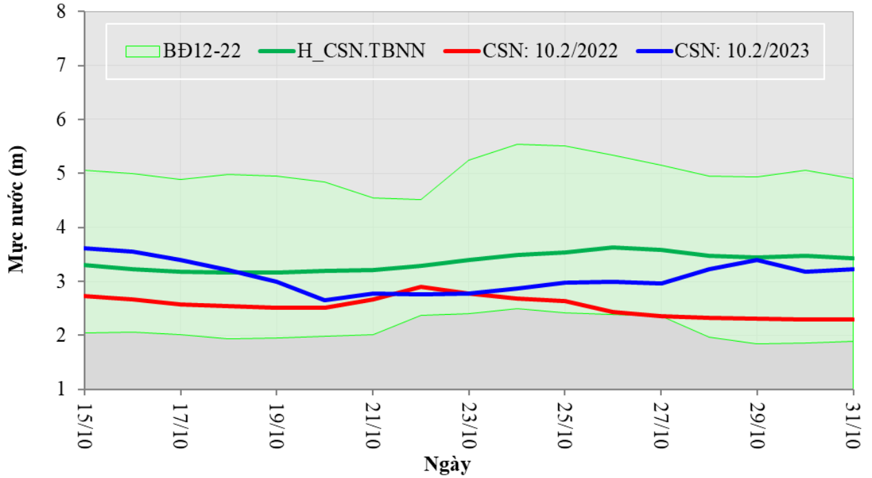
Hình 1. Diễn biến mực nước tại trạm Chiềng Sẻn trong nửa cuối tháng 10/2023
