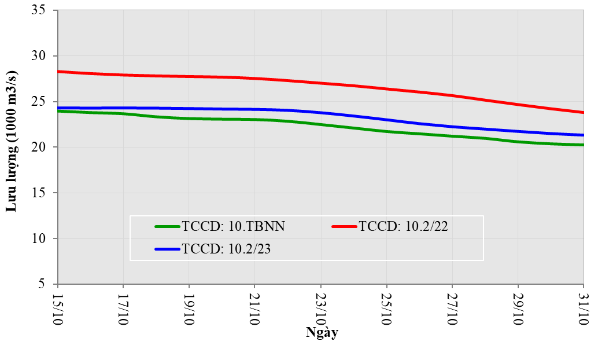
Hình 10. Diễn biến lưu lượng của hai trạm Tân Châu và Châu Đốc nửa cuối tháng 10/2023
