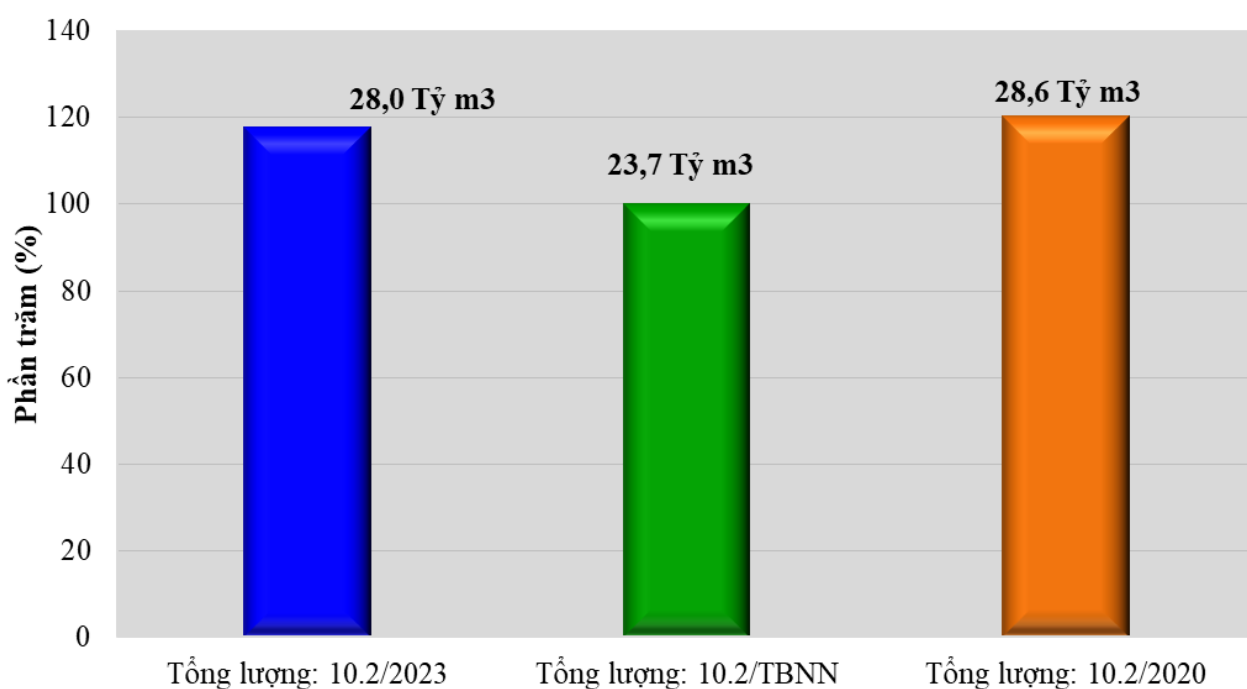
Hình 6. Tổng lượng dòng chảy tại trạm Kra-chê trong nửa cuối tháng 10/2023
