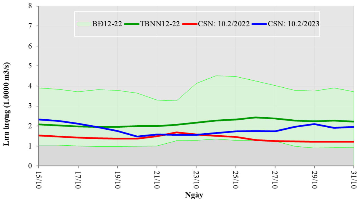
Hình 2. Diễn biến dòng chảy tại trạm Chiềng Sẻn trong nửa cuối tháng 10/2023
