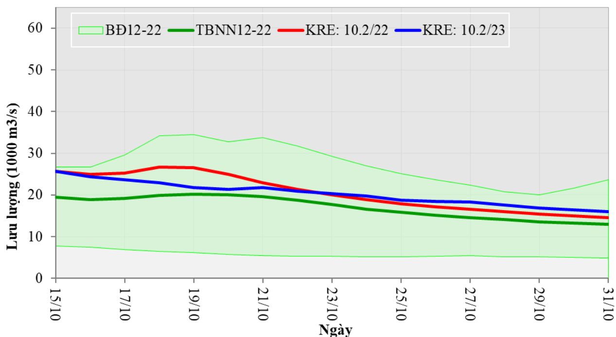
Hình 5. Diễn biến lưu lượng tại trạm Kra-chê trong nửa cuối tháng 10/2023
