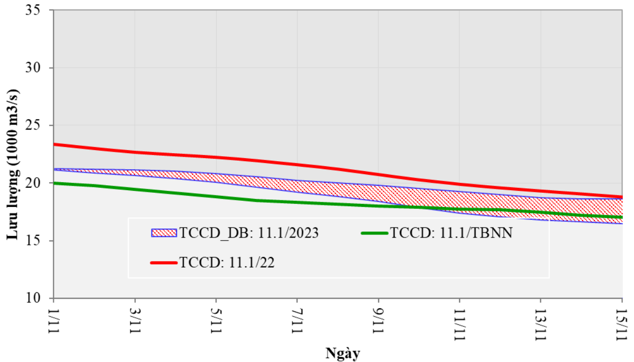
Hình 13. Dự báo lưu lượng tới hai trạm Tân Châu và Châu Đốc trong nửa đầu tháng 11/2023
