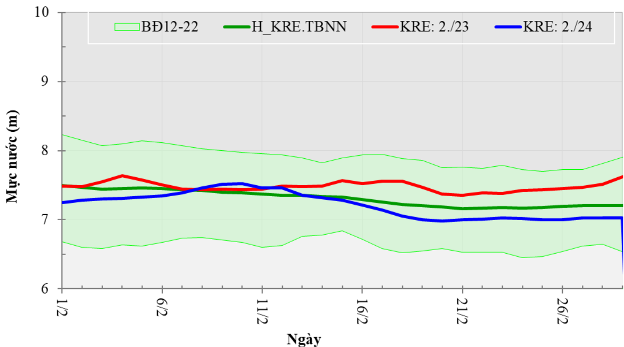
Hình 4. Diễn biến mực nước tại trạm Kra-chê trong tháng 02/2024
