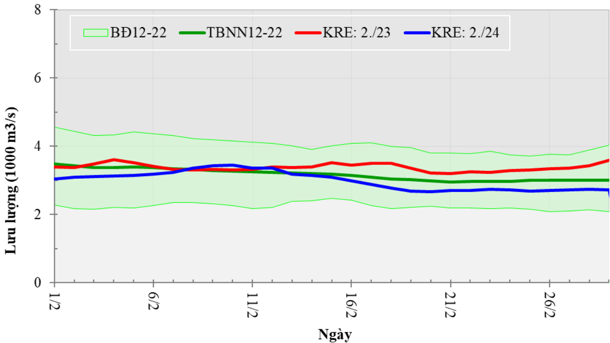
Hình 5. Diễn biến lưu lượng tại trạm Kra-chê trong tháng 02/2024
