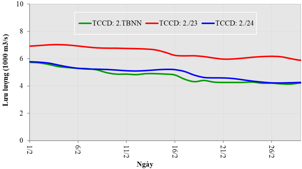
Hình 10. Diễn biến lưu lượng qua hai trạm Tân Châu và Châu Đốc tháng 02/2024
