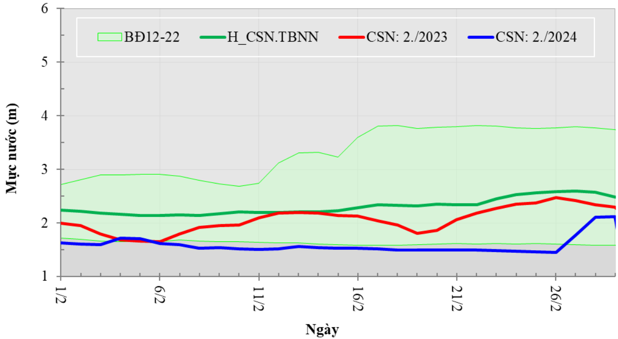
Hình 1. Diễn biến mực nước tại trạm Chiềng Sẻn trong tháng 02/2024
