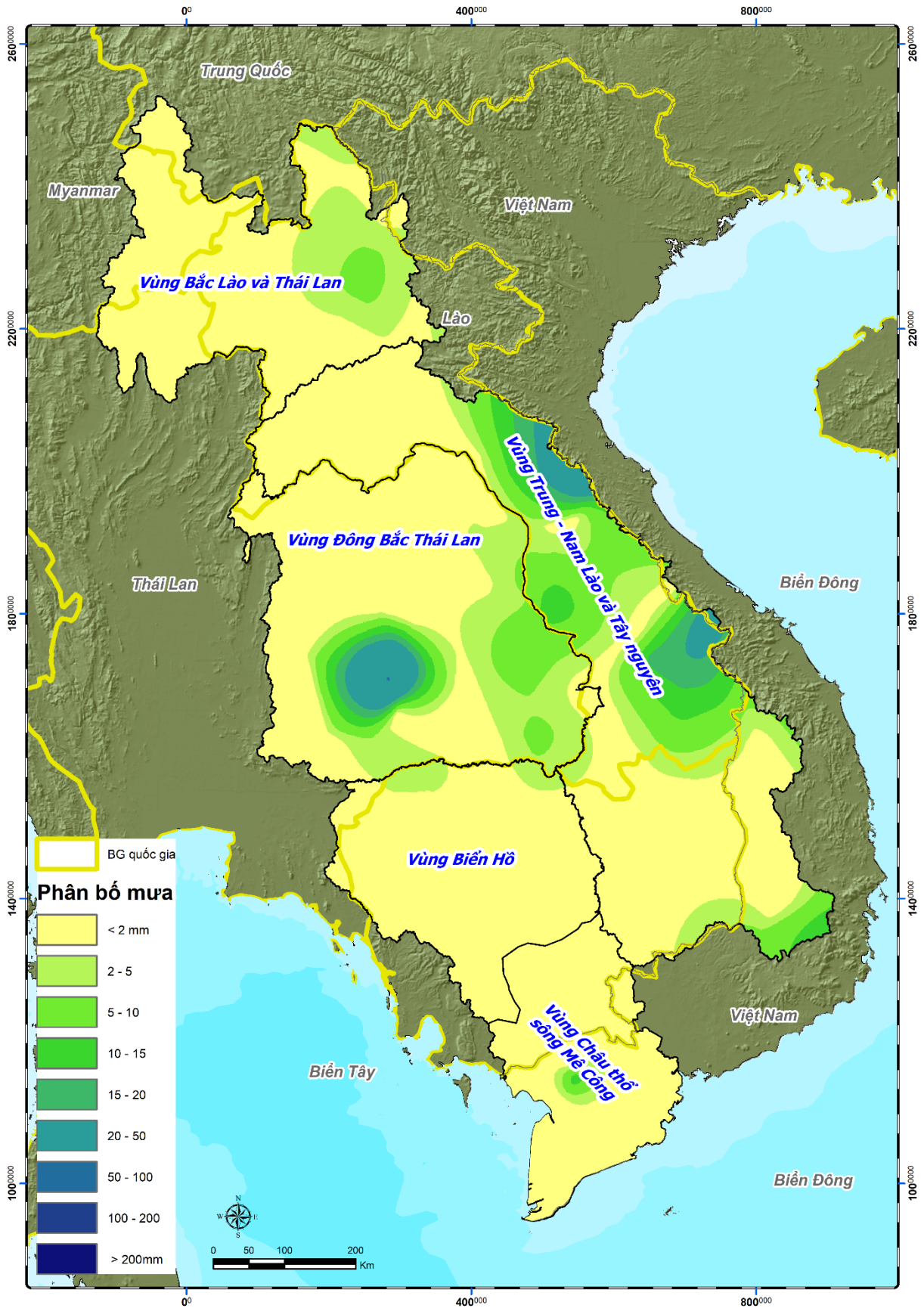
Bản đồ 2. Bản đồ phân bố mưa vùng hạ lưu vực Mê Công tháng 02/2024
