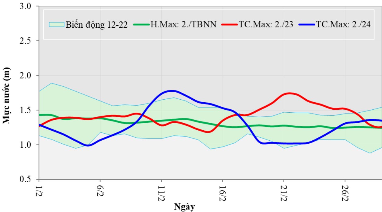
Hình 9. Diễn biến mực nước lớn nhất ngày tại trạm Tân Châu tháng 02/2024
