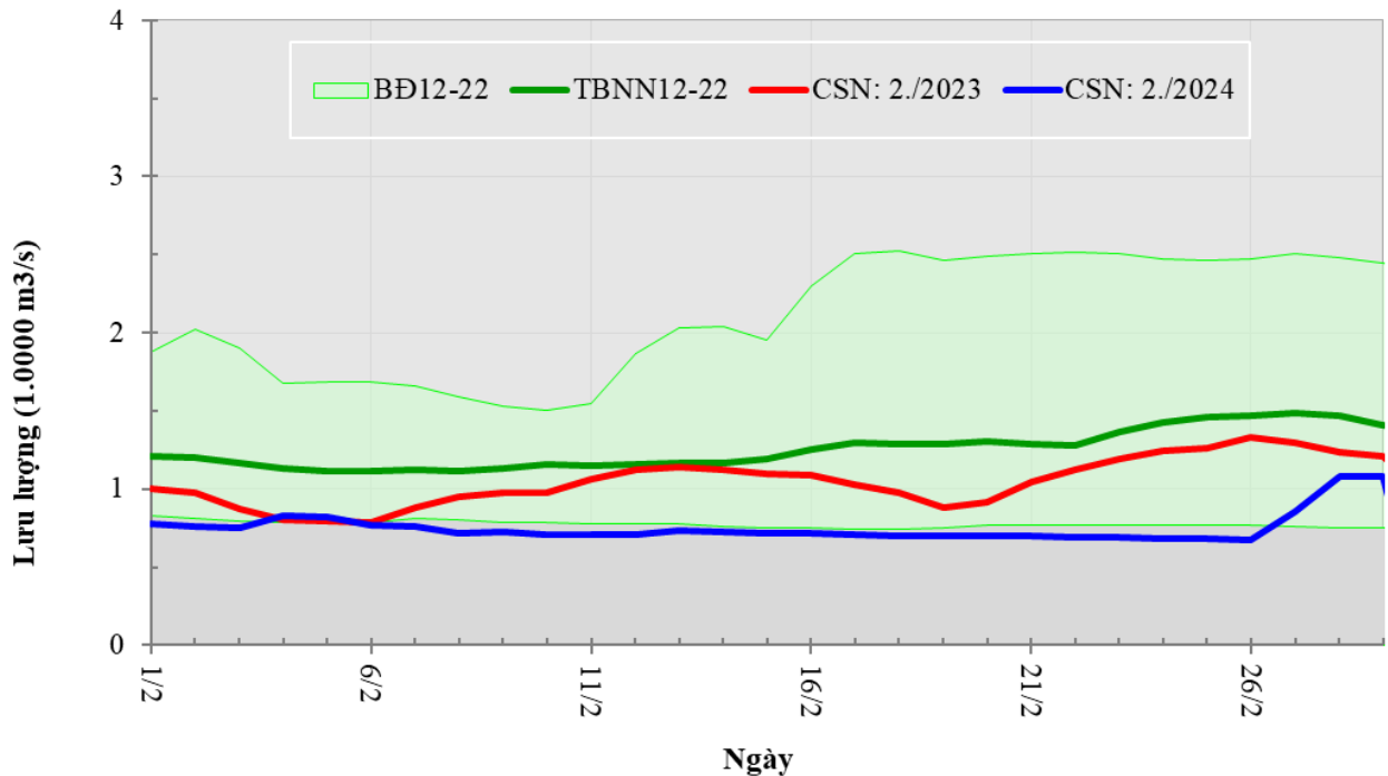
Hình 2. Diễn biến dòng chảy tại trạm Chiềng Sẻn trong tháng 02/2024
