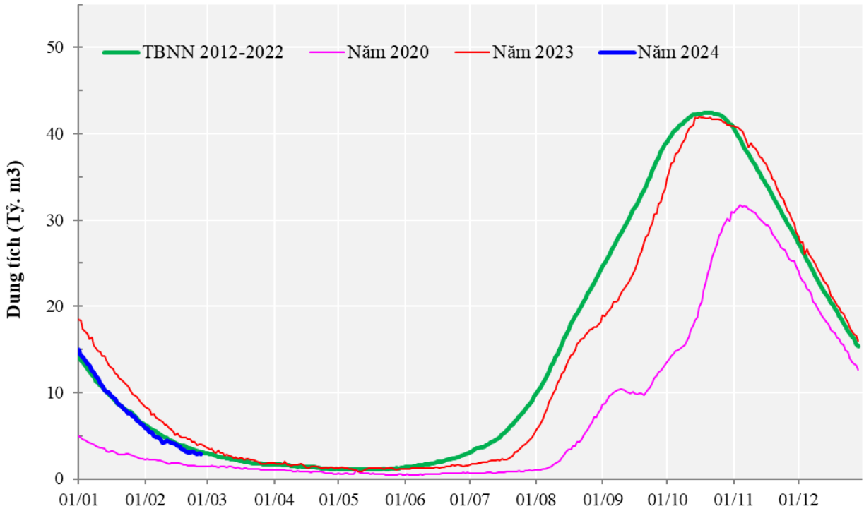
Hình 8. Diễn biến dung tích Biển Hồ tính đến cuối tháng 02/2024
