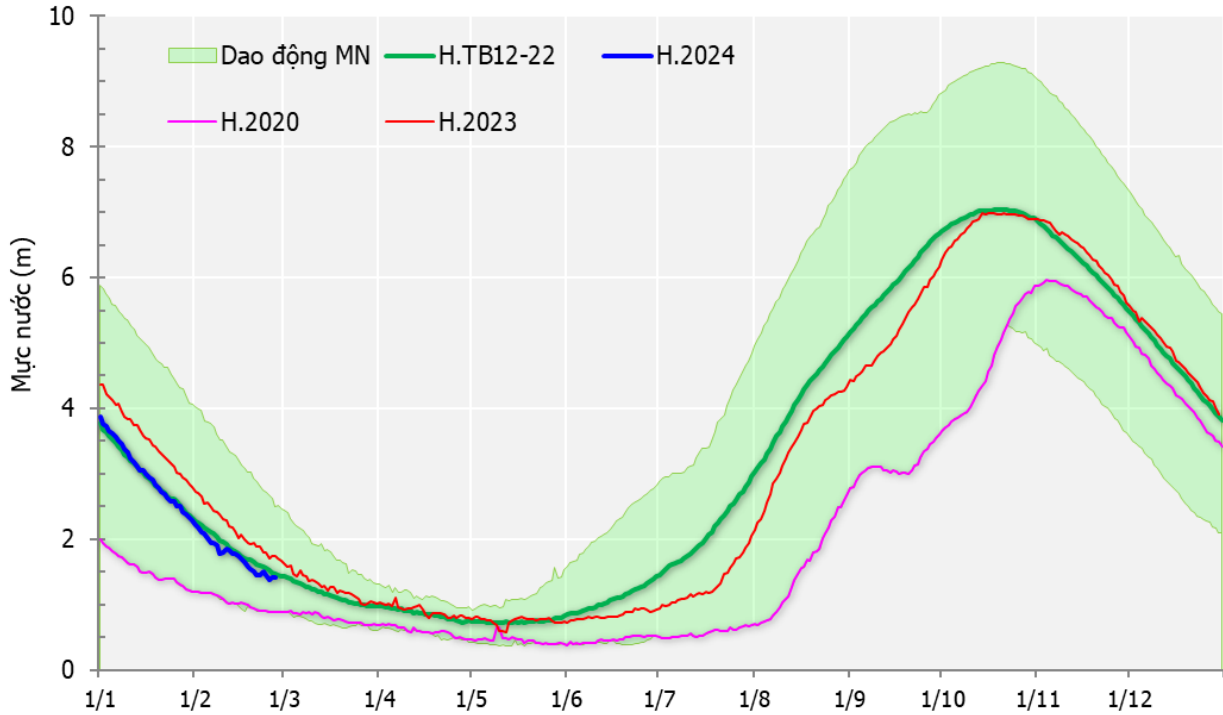
Hình 7. Diễn biến mực nước Biển Hồ tính đến cuối tháng 02/2024
