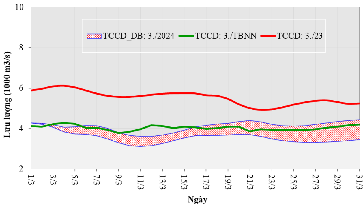
Hình 13. Dự báo lưu lượng tới hai trạm Tân Châu và Châu Đốc trong tháng 3/2024
