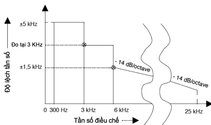
Hình 1. Độ lệch tần số theo tần số điều chế
