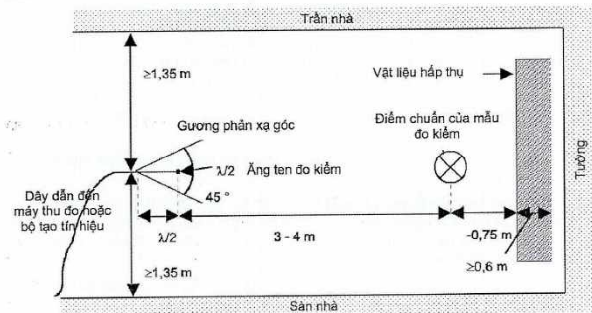
Hình C.2 - Bố trí vị trí đo trong nhà
