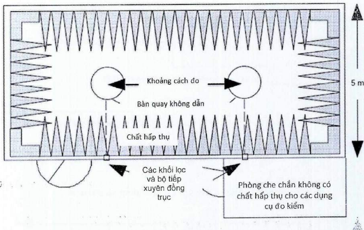
Hình A.4 - Ví dụ về cấu trúc của phòng đo không đội được che chắn
