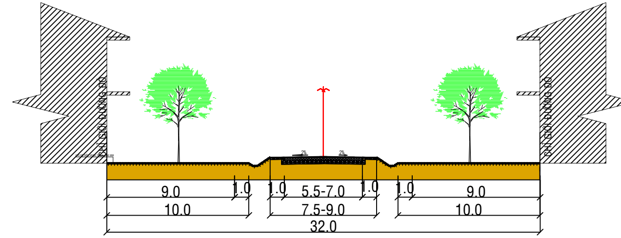
ẢNH MINH HỌA VỀ ĐỘ VƯỢN BAN CÔNG LỘ GIỚI, TẦNG CAO VÀ CAO ĐỘ XÂY DỰNG
